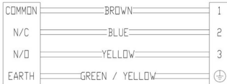
MICROSWITCH
