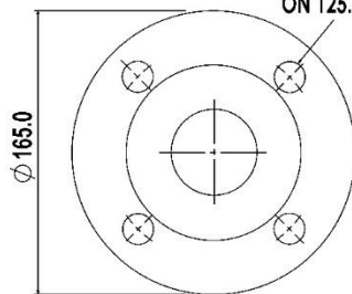
50mm PIPE FLANGE TO BS EN 1092-1 PN16
