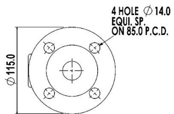
25mm PIPE FLANGE ADAPTOR TO BS EN 1092-1 PN16
