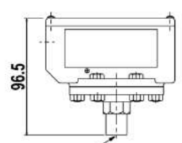
25mm PIPE FLANGE ADAPTOR TO BS EN 1092-1 PN16
